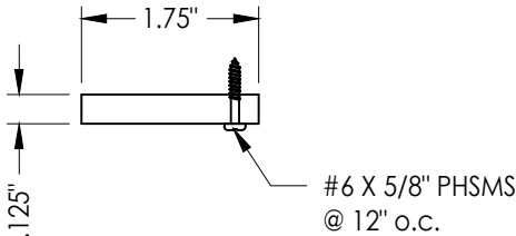
6 ASTRAGAL
